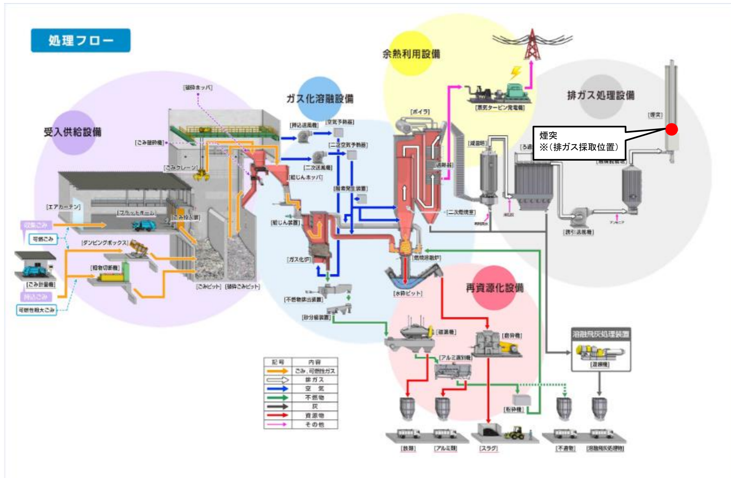
エネルギー回収施設(立谷川)における排ガスの採取位置図
